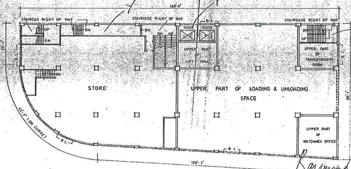
Cockloft Plan
