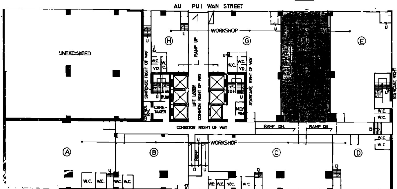
GRD. FL. PL. (1:400)
